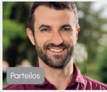
Marcel Siegenthaler
