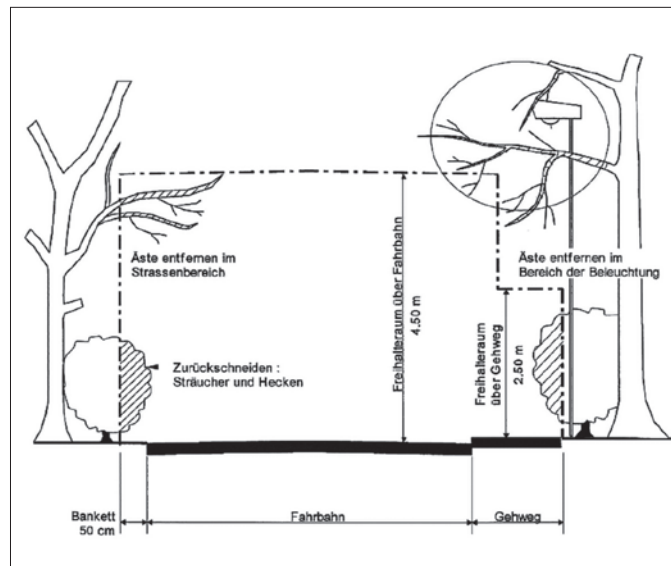
Das nach Strassen-gesetz vorgeschriebene Lichttraumprofil.
