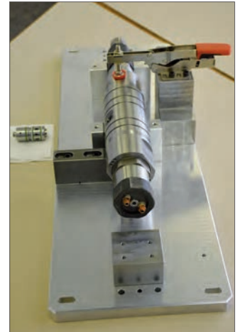
Der bei DUAP neu entwickelte DUAGAS- & Wasserstoff-DI-Injektor.
